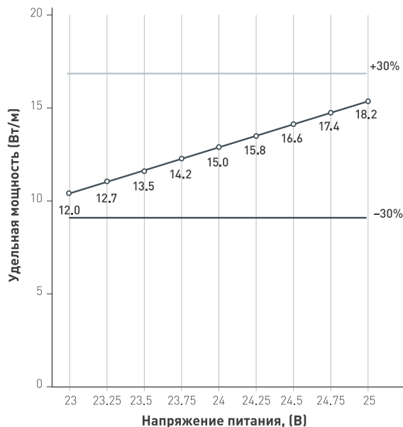
Зависимость удельной мощности ленты от напряжения питания*
