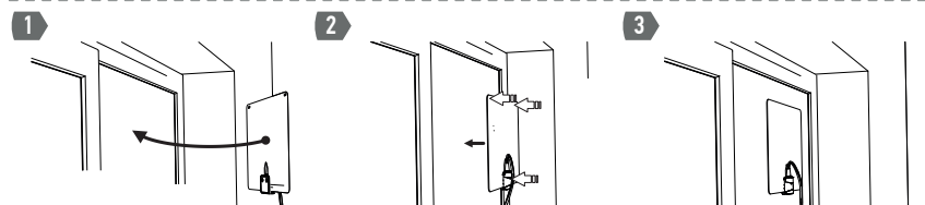
Установка на оконное стекло
