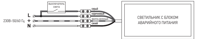
Рис.1. 230В шамчыракты токко туташтыруу схемасы
