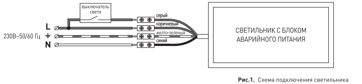
Рис.1. Схема подключения светильника
