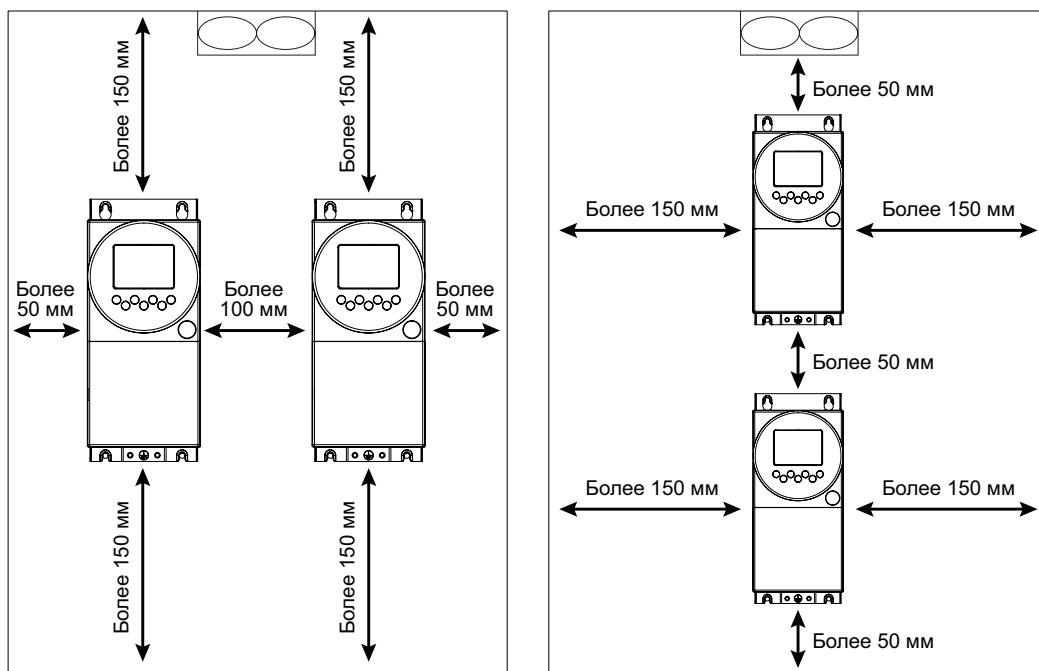
Рекомендованный способ установки: горизонтально
