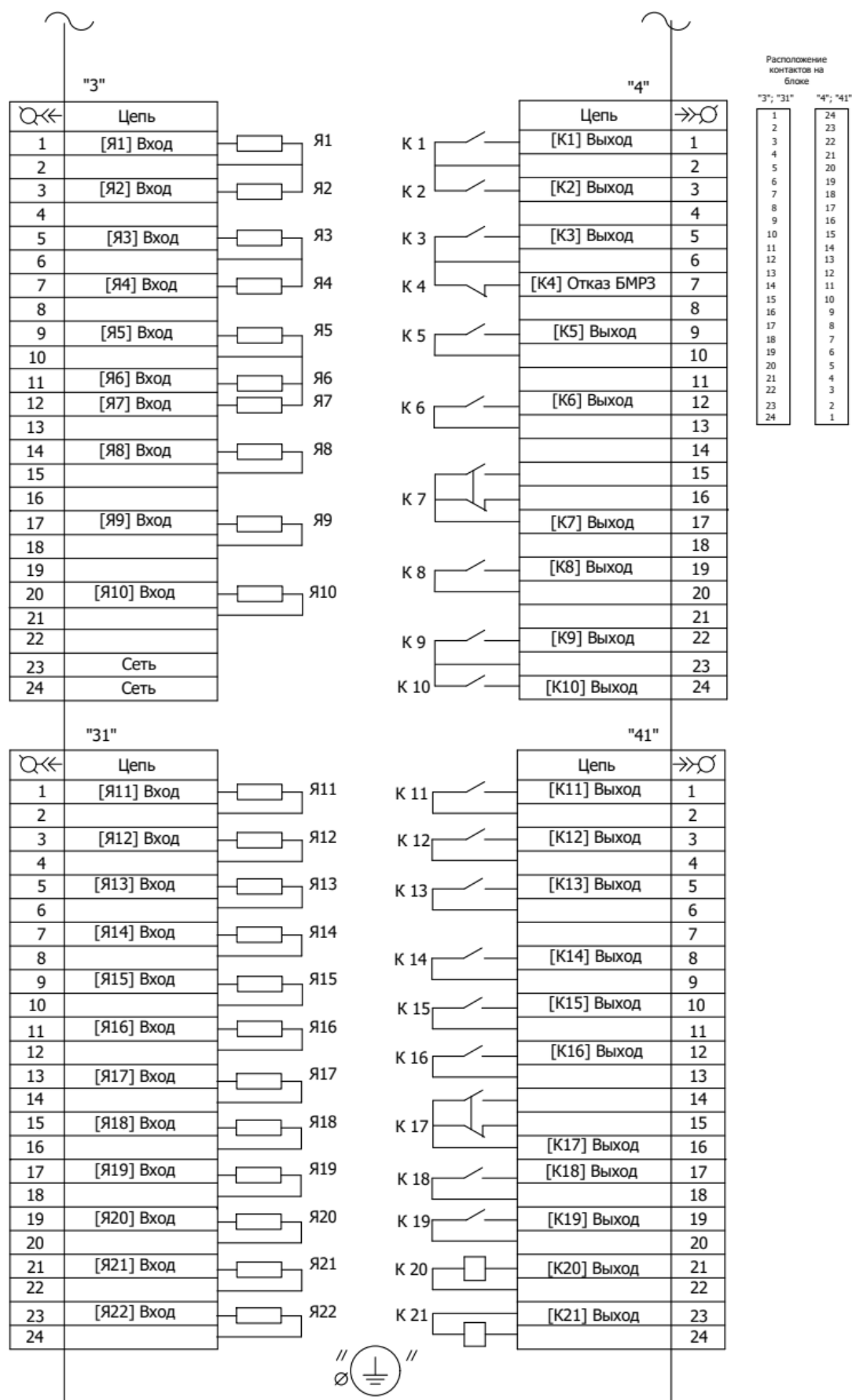
Рисунок А.3 - Схема электрическая подключения дискретных входов и выходов БФПО
