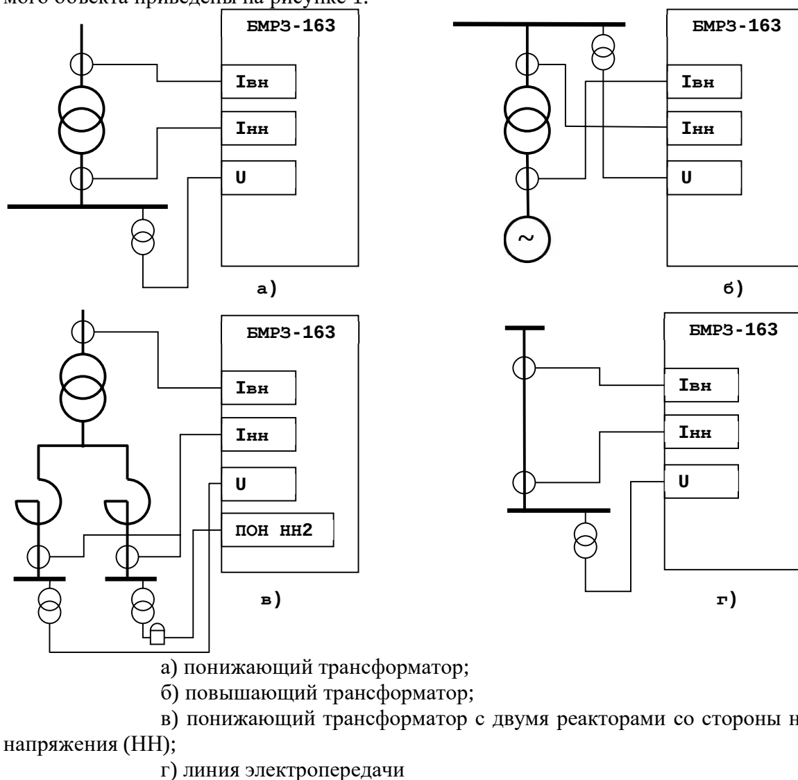
Рисунок 1 - Примеры подключения измерительных цепей
