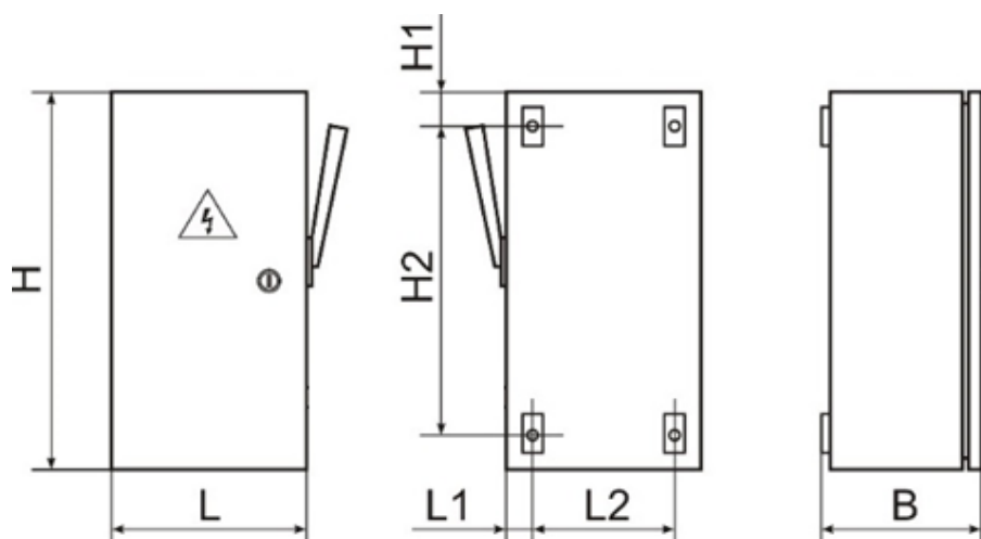
Рисунок 1. Общий вид и габаритные размеры ЯРП11М-3
