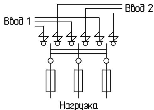
Рисунок 4. Схема электрическая принципиальная ЯРП11М-7
