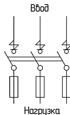
Рисунок 2. Схема электрическая принципиальная ЯРП11М-3
