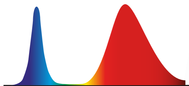
Красно-синий спектр
