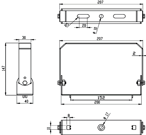
Рисунок 1. Габаритные размеры поворотного кронштейна для накладного монтажа светильников SPP-402
