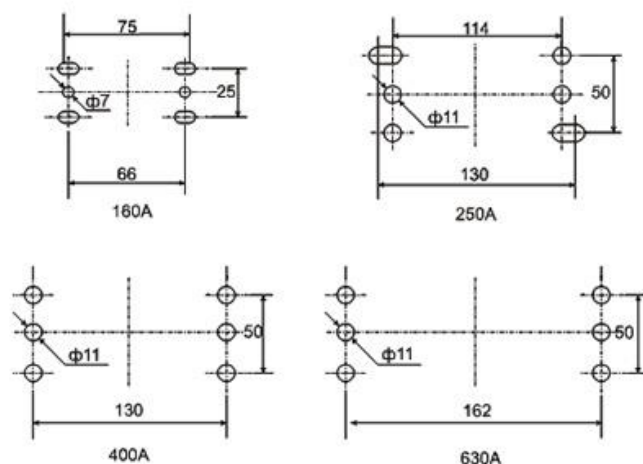
Рисунок 2. Установочные размеры.
