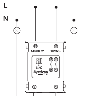
Двухполюсный ВЫКЛЮЧАТЕЛЬ
