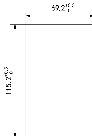
Рисунок 6.1b). Чертеж установки панели управления (вырез в двери шкафа)
