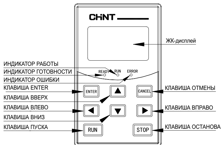
Рисунок 6.1a). Внешний вид панели управления
