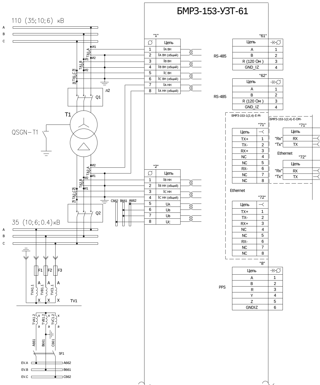
Рисунок А.1 - Схема электрическая подключения при использовании трех ТТ со стороны НН
