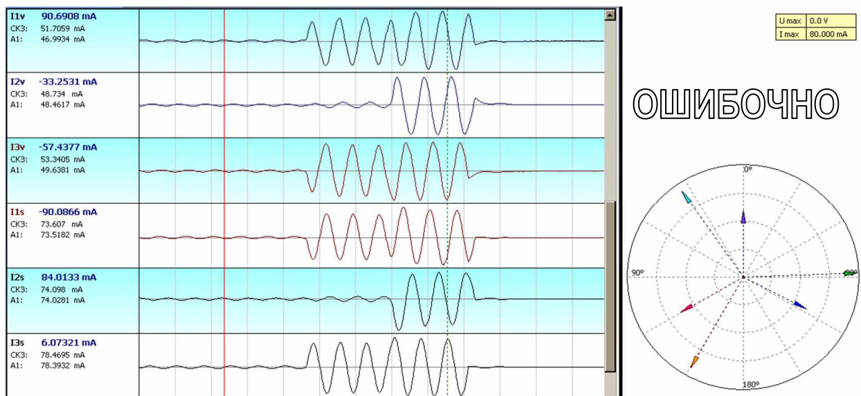
Рисунок Е.5 - Неправильная фазировка и выравнивание токов циркуляции в доаварийном режиме
