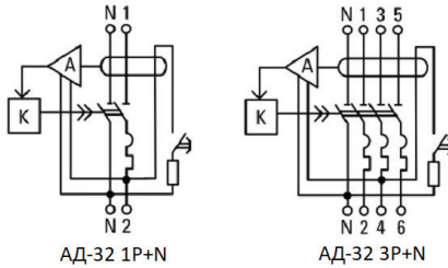
Рисунок 1 – Принципиальная схема электрическая АД-32
