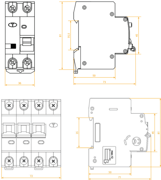
Рисунок 2 – Габаритные размеры АДВТ
