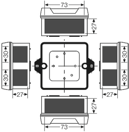
Стенки корпуса
