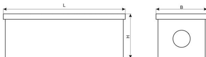
Рисунок 1. Общий вид и габаритные размеры поста управления кнопочного в металлическом корпусе
