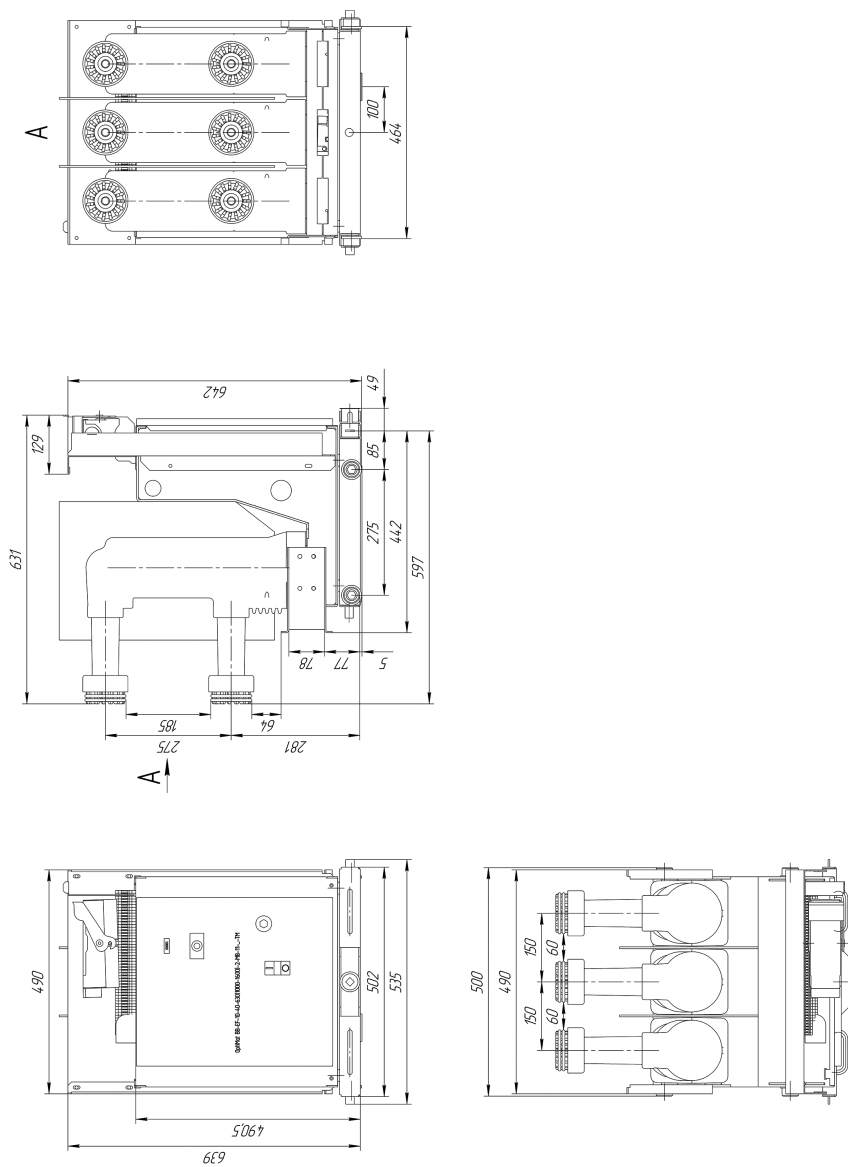
Рисунок В.1.7 – OptiMat BB-EF-10-40-630 (1000-1600)-2-MB-11
