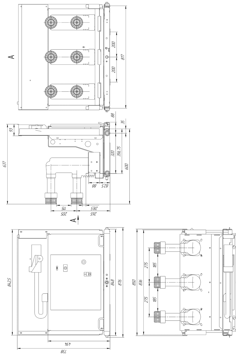
Рисунок В.1.27 – OptiMat BB-EF-10-20(25;31.5;40)-630(1000-1600)-4-MB-30
