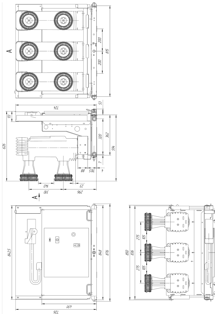
Рисунок В.1.12 – OptiMat-BB-EF-10-50-2500-2-MB-30
