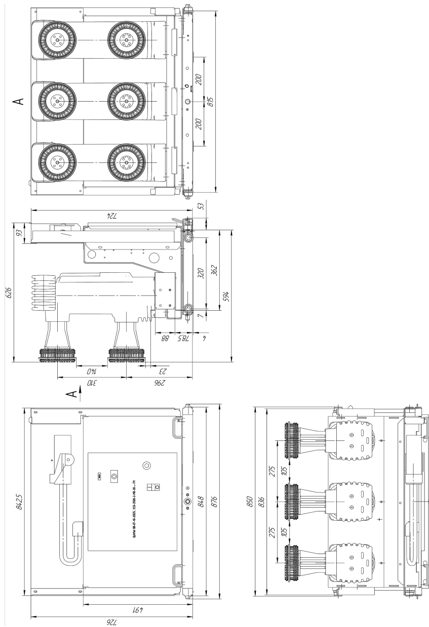
Рисунок В.1.4 – OptiMat BB-EF-10-20(25;31.5) – 2500-2-MB-30
