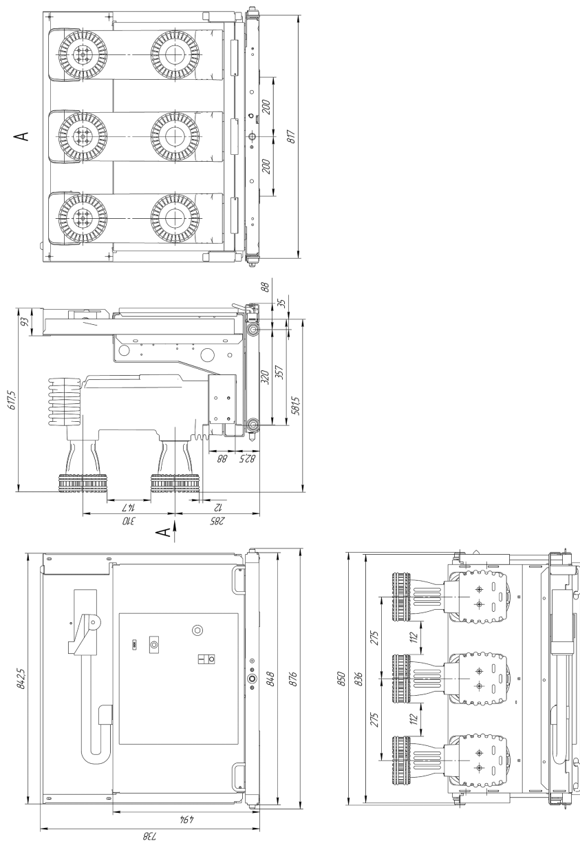
Рисунок В.1.31 – OptiMat BB-EF-10-20(25;31;5;40)-3150(4000)-4-MB-30
