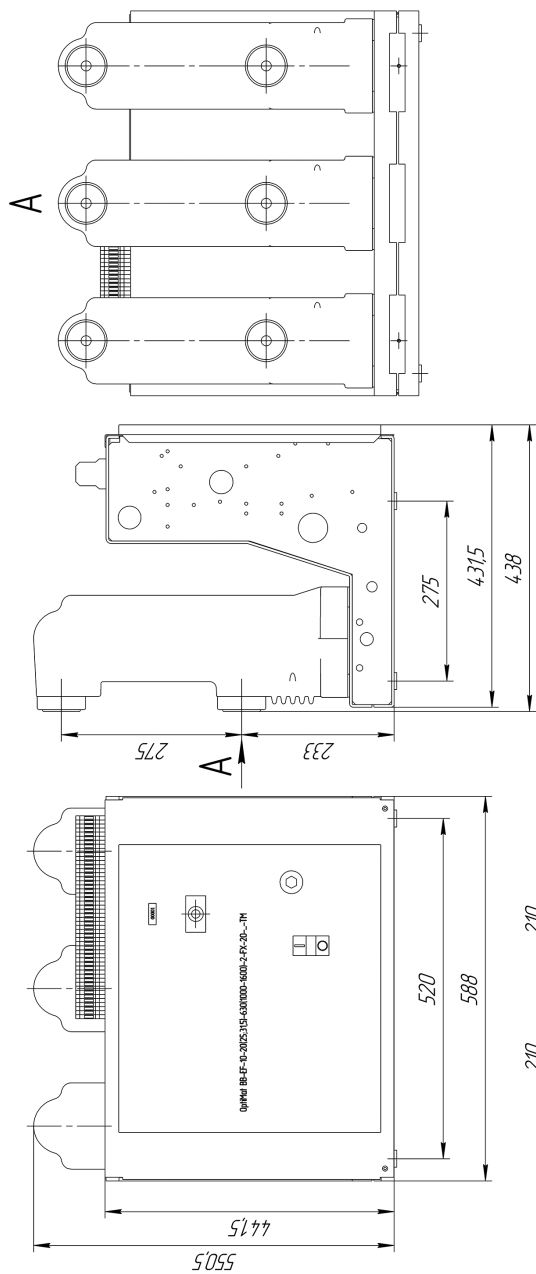
Рисунок А.2 – OptiMat BB-EF-10-20(25;31.5)– 630(1000-1600)-2-FX-20
