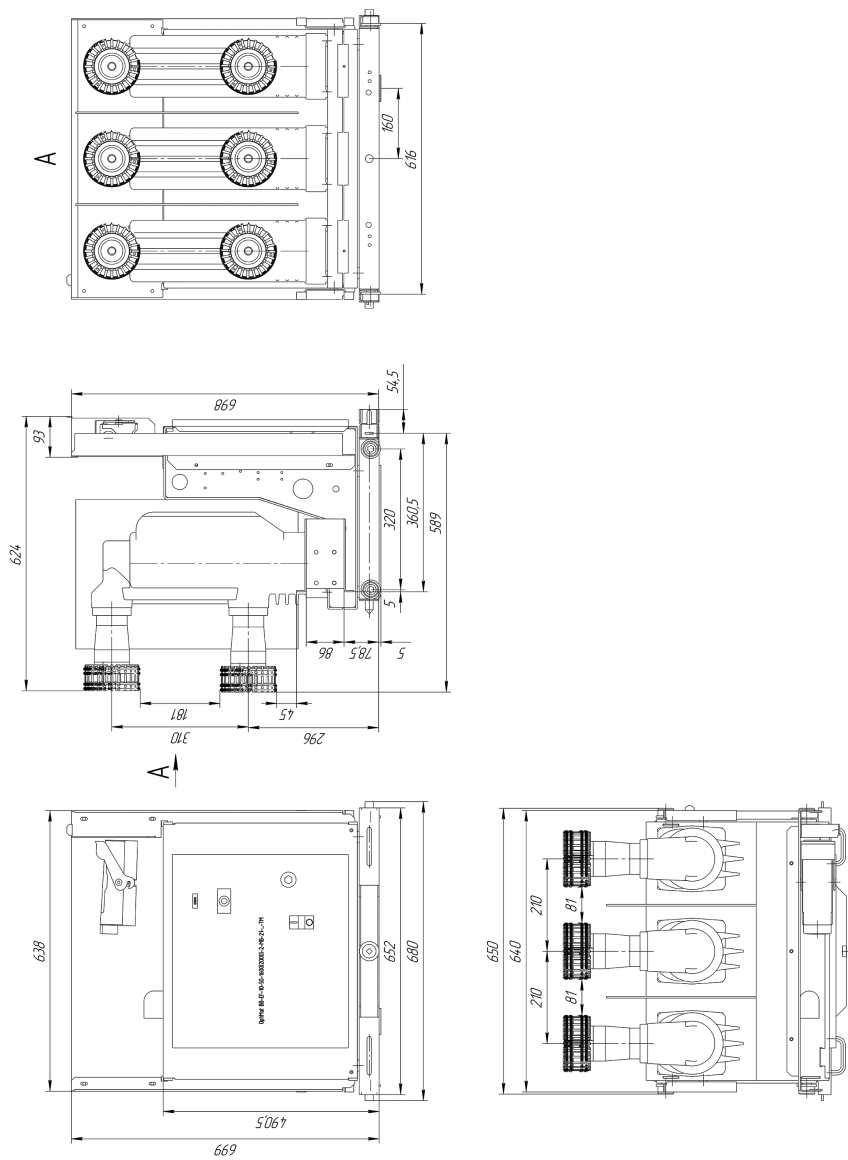
Рисунок В.1.11 – OptiMat BB-EF-10-50-1600(2000)-2-MB-21
