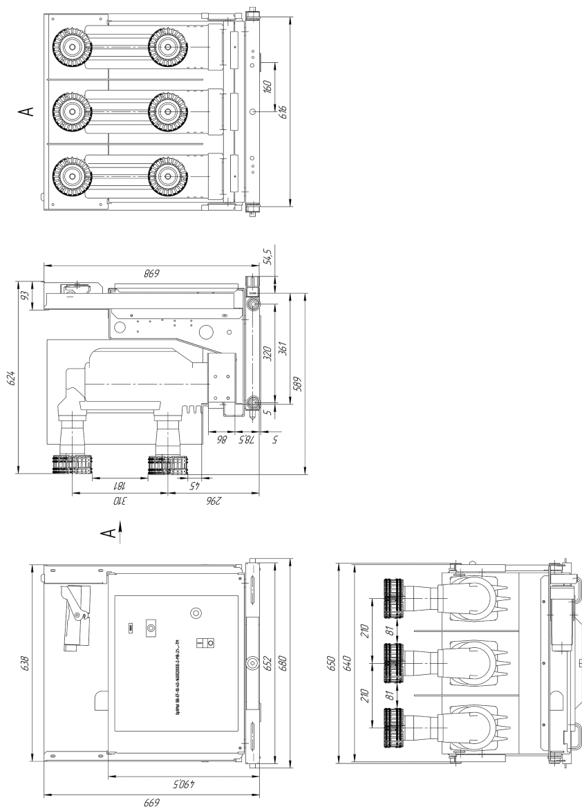
Рисунок В.1.9 – ОптіMat BB-EF-10-40-1600(2000)-2-MB-21
