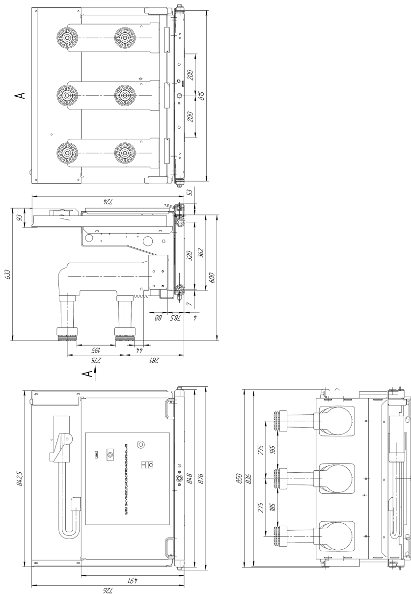
Рисунок В.1.1.5 – OptiMat BB-EF-10-20(25;31.5;40;50) – 630(1000-1600) – 2-МВ-30
