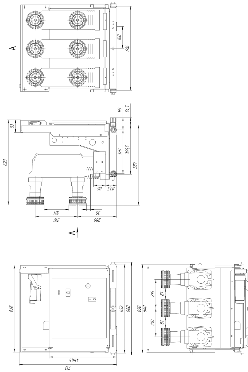
Рисунок В.1.28 – OptiMat BB-EF-10-20(25;31.5;40)-1600(2000)-4-MB-20
