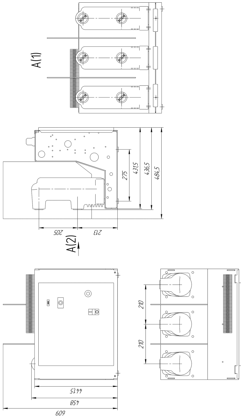
Рисунок А.25 – OptiMat BB-EF-10-20(25;31.5;40)-630(1000-1600)-4-FX-21
