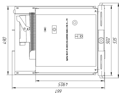
Рисунок В.1.1 – OptiMat BB-EF-10-20(25;31.5)-630 (1000-1600)-2-МВ-11
