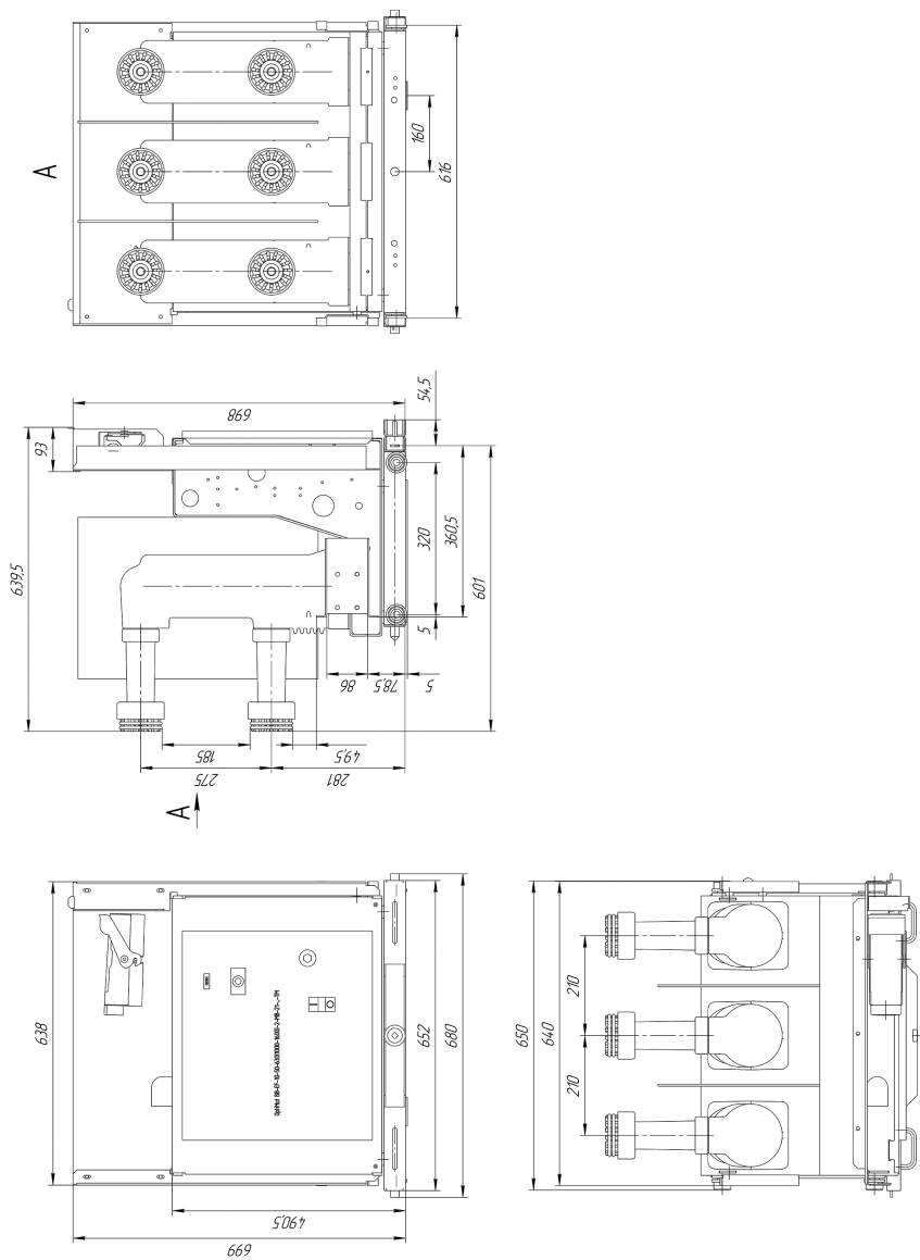
Рисунок В.1.13 – OptiMat BB-EF-10-50-630(1000-1600)-2-MB-21
