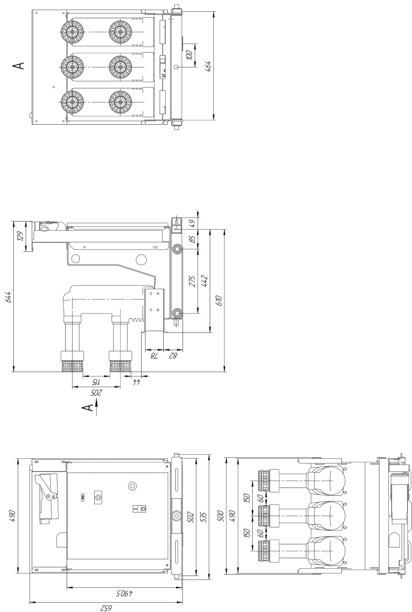
Рисунок В.1.25 – OptiMat ВВ-ЕF-10-20(25;31;5;40)-630(1000-1600)-4-МВ-10
