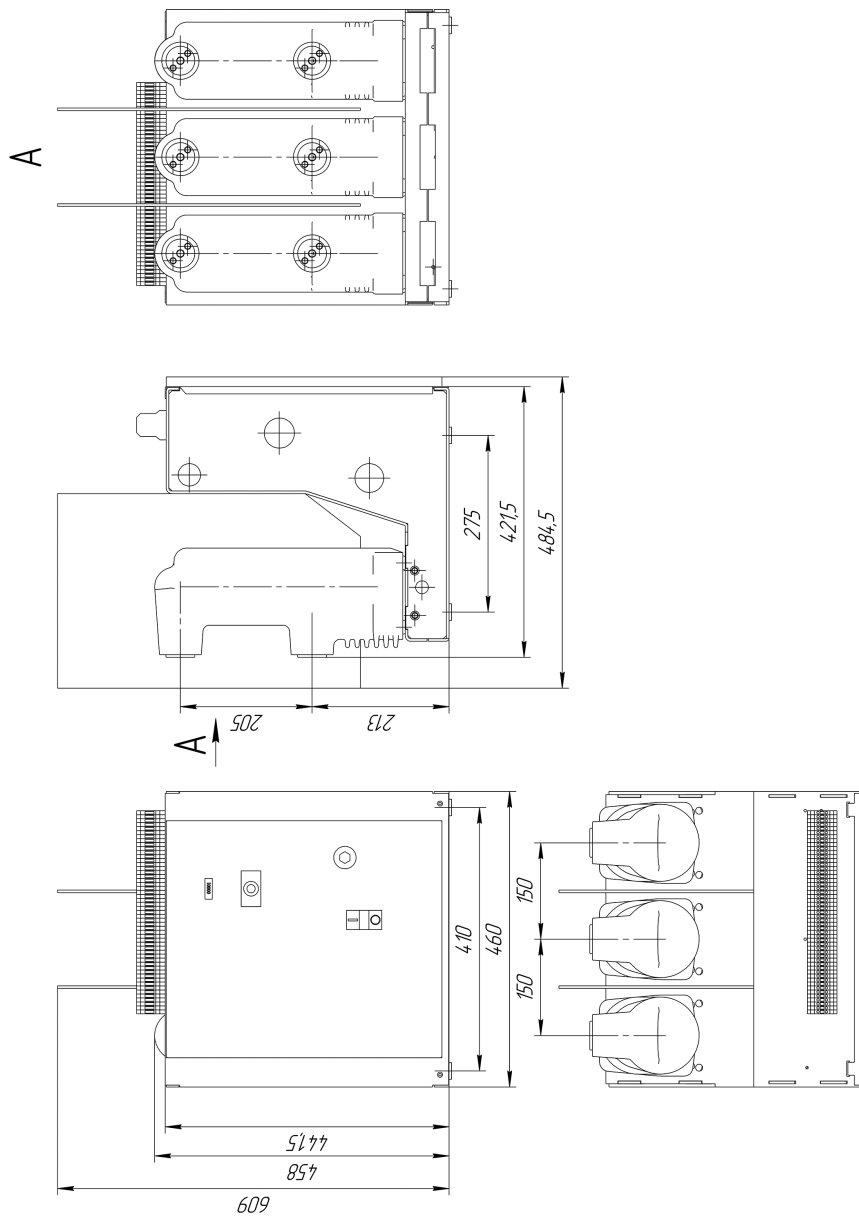
Рисунок А.24 – Опрыскатель ВВ-ЕФ-10-20(25;31;5;40)-630(1000-1600)-4-FX-11
