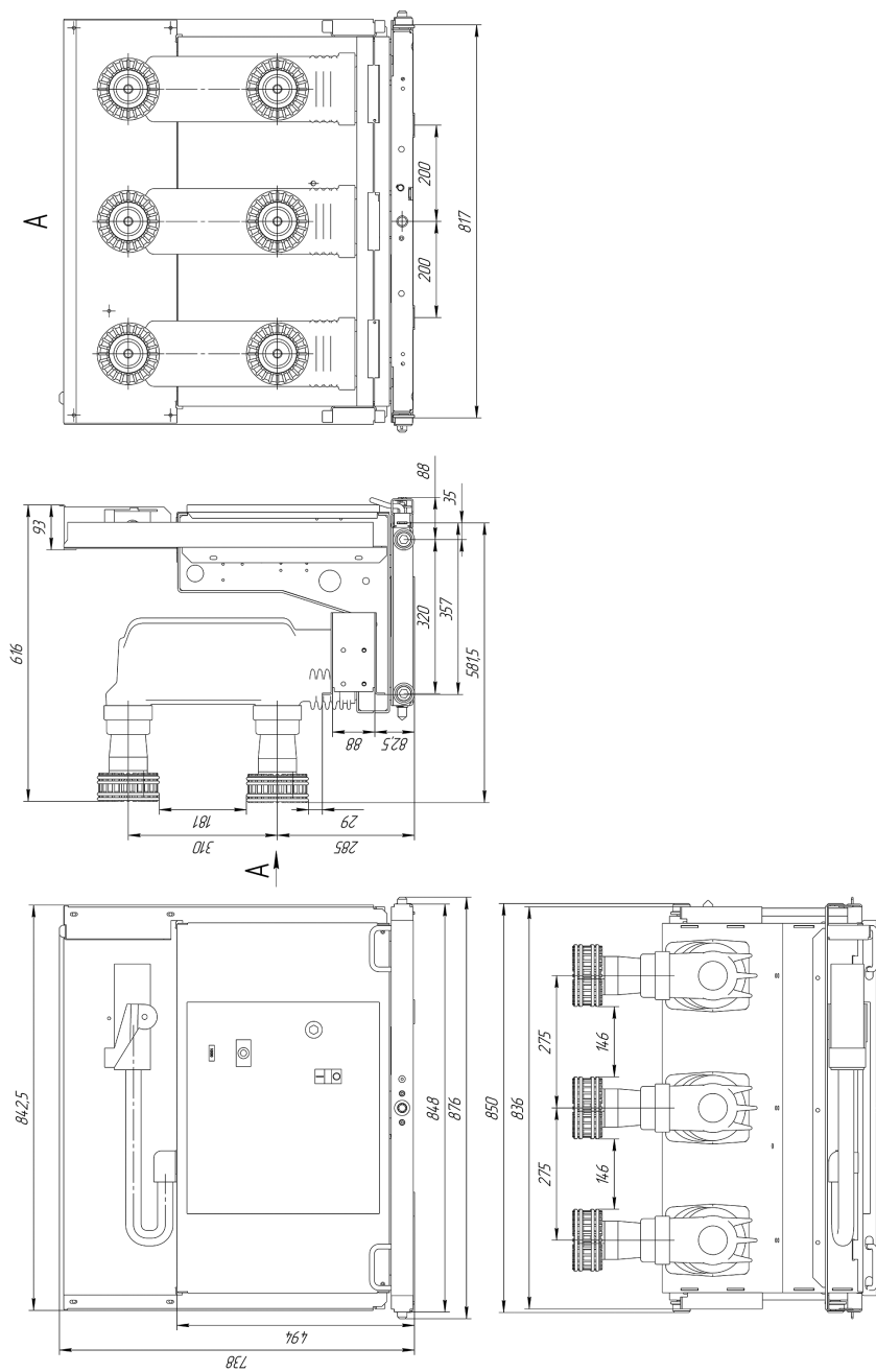
Рисунок В.1.29 – OptiMat-BB-EF-10-20(25;31.5;40)-1600(2000)-4-MB-30
