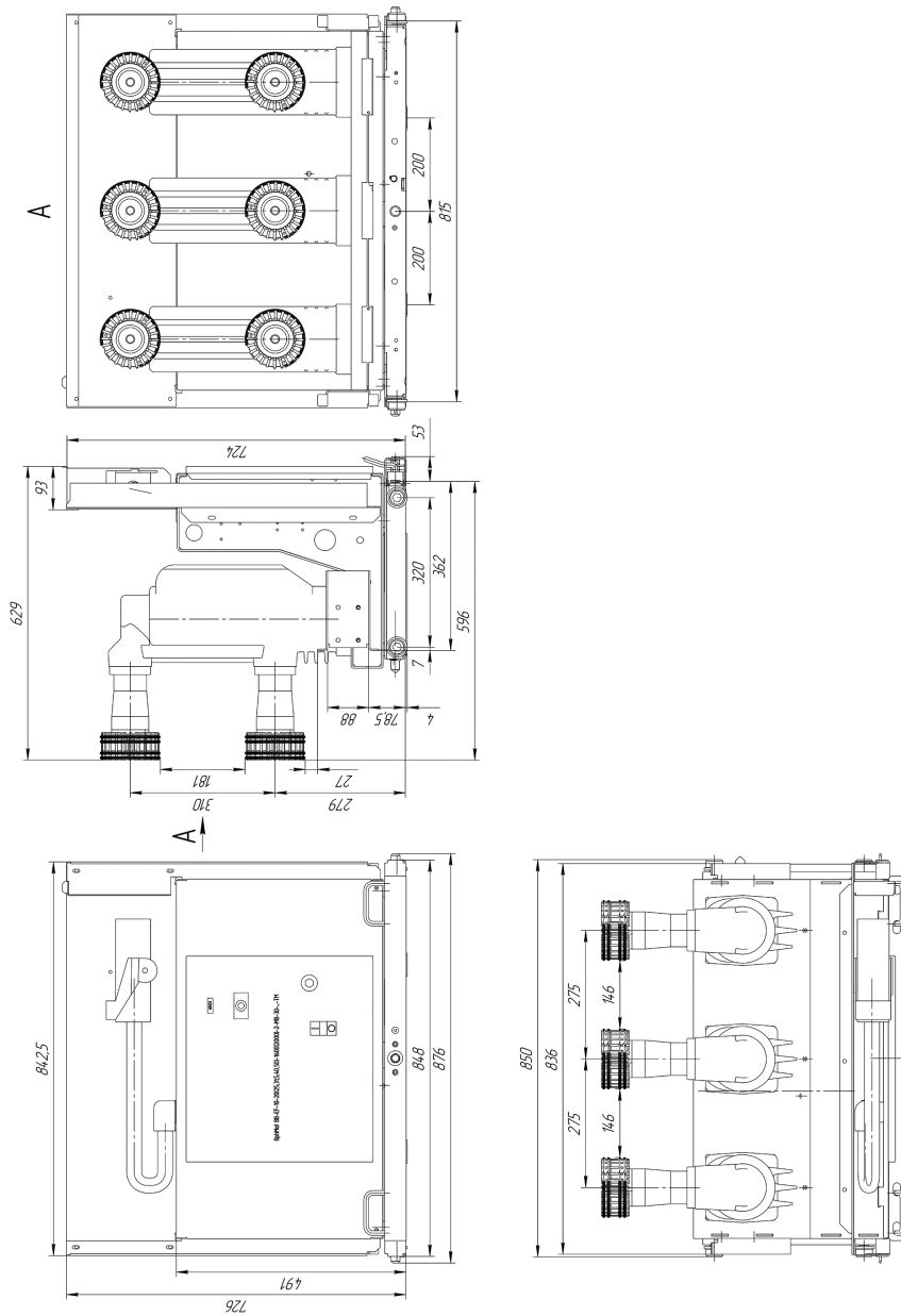
Рисунок В.1.6 – OptiMat BB-EF-10-20(25;31.5;40;50) -1600(2000) -2-MB-30
