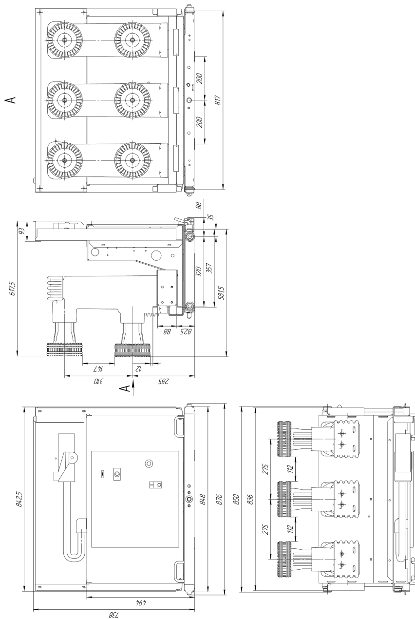
Рисунок В.1.30 – OptiMat BB-EF-10-20(25;31.5;40)-2500-4-MB-30
