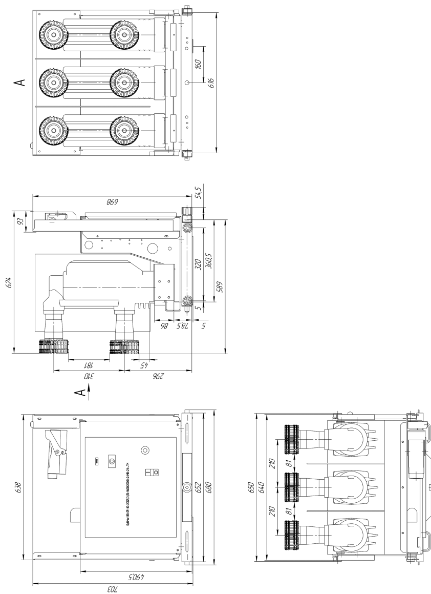
Рисунок В.1.3 – OptiMat BB-EF-10-20(25;31.5)- 1600(2000)-2-MB-21
