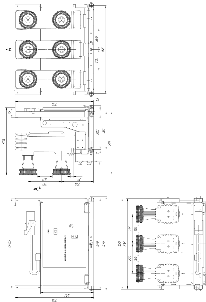
Рисунок В.1.15 – OptiMat BB-EF-10-40-3150(4000)-2-MB-30
