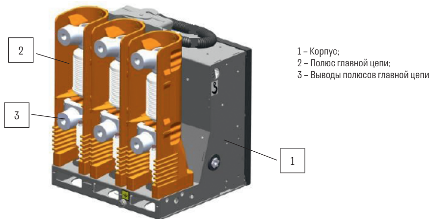
Рисунок 1.1 – Общий вид выключателя со сборной изоляцией.
