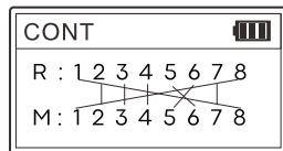
Контакты 5 и 6 перекрестно соединены, контакты 1 и 8 перекрестно соединены
