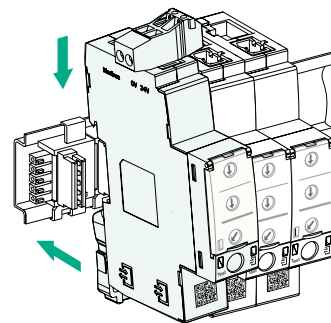
До 12 модулей IFM в ряд
