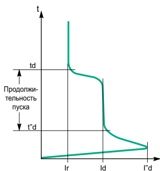
Типовая пусковая характеристика электродвигателя
