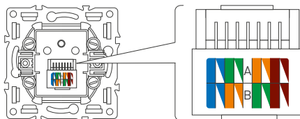
Рис. 1. Схема подключения
