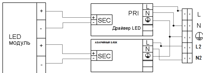
Светильник с аварийным блоком.
