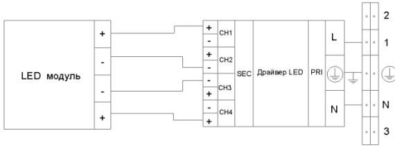
Мал. 2. Схема електричних з'єднань:
