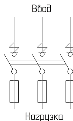
Рисунок 2. Схема электрическая принципиальная ЯРП
