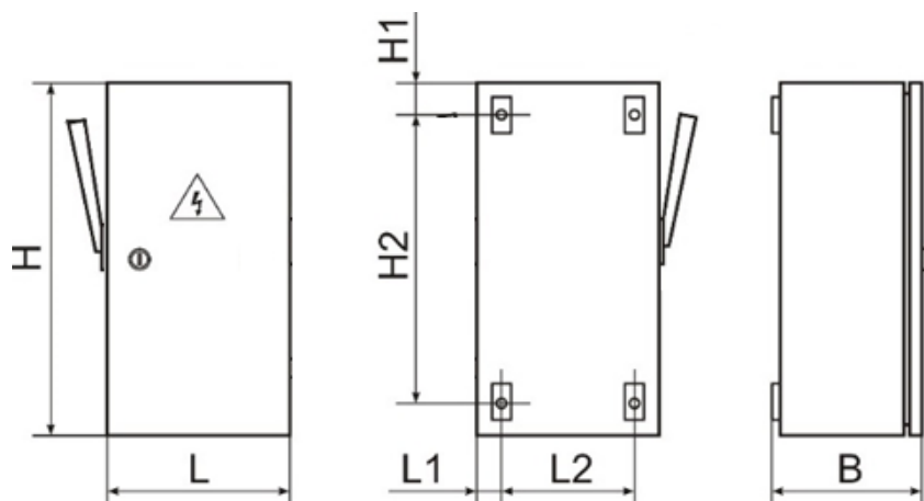
Рисунок 3. Общий вид и габаритные размеры ЯРПП
