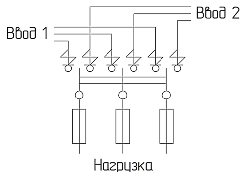
Рисунок 4. Схема электрическая принципиальная ЯРПП
