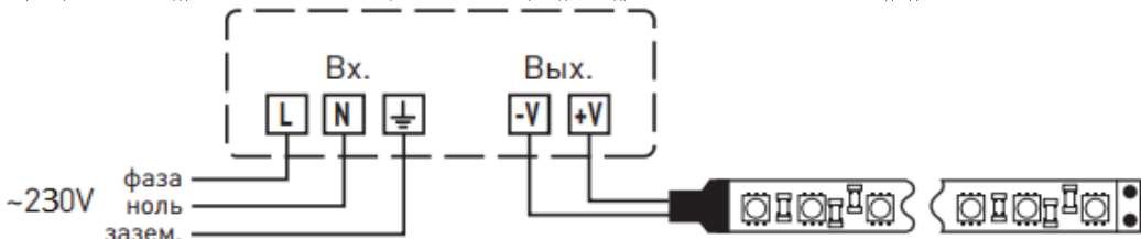
Рисунок 1 – Схема подключения
