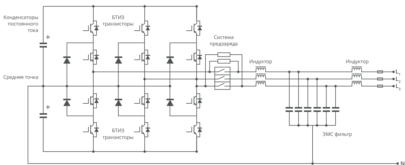
Принципиальная схема топологии трехуровневого инвертора
