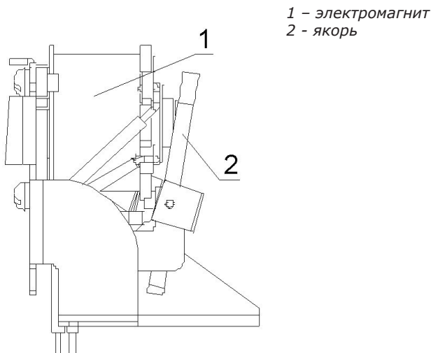
Рисунок 3 – Независимый расцепитель.
