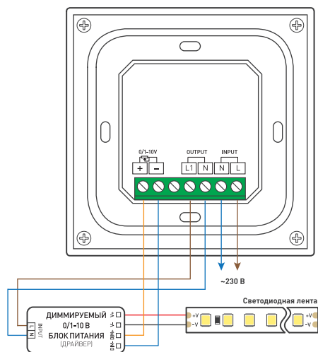
Рисунок 2. Схема подключения панели Rotary SMART-P96-DIM White с использованием выхода «AC OUT»
