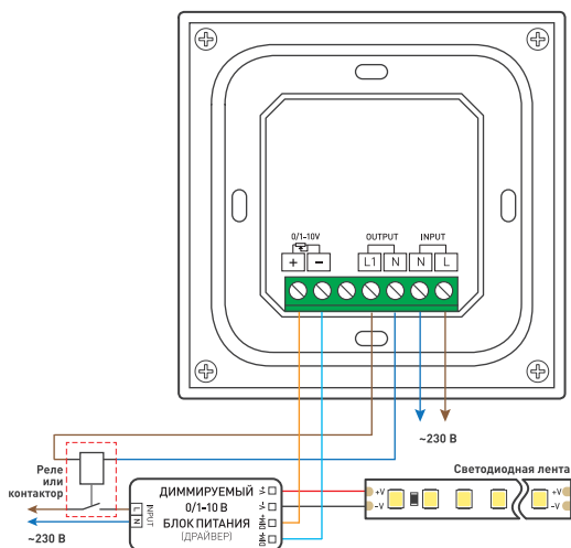
Рисунок 3. Схема подключения панели Rotary SMART-P96-DIM White с использованием коннектора или реле
