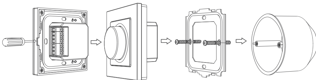
Рисунок 4. Монтаж панели Rotary SMART-P96-DIM White
