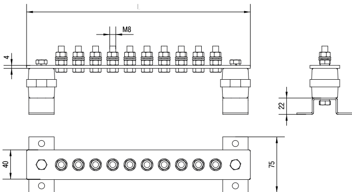
Рисунок 1 – Габаритные размеры
