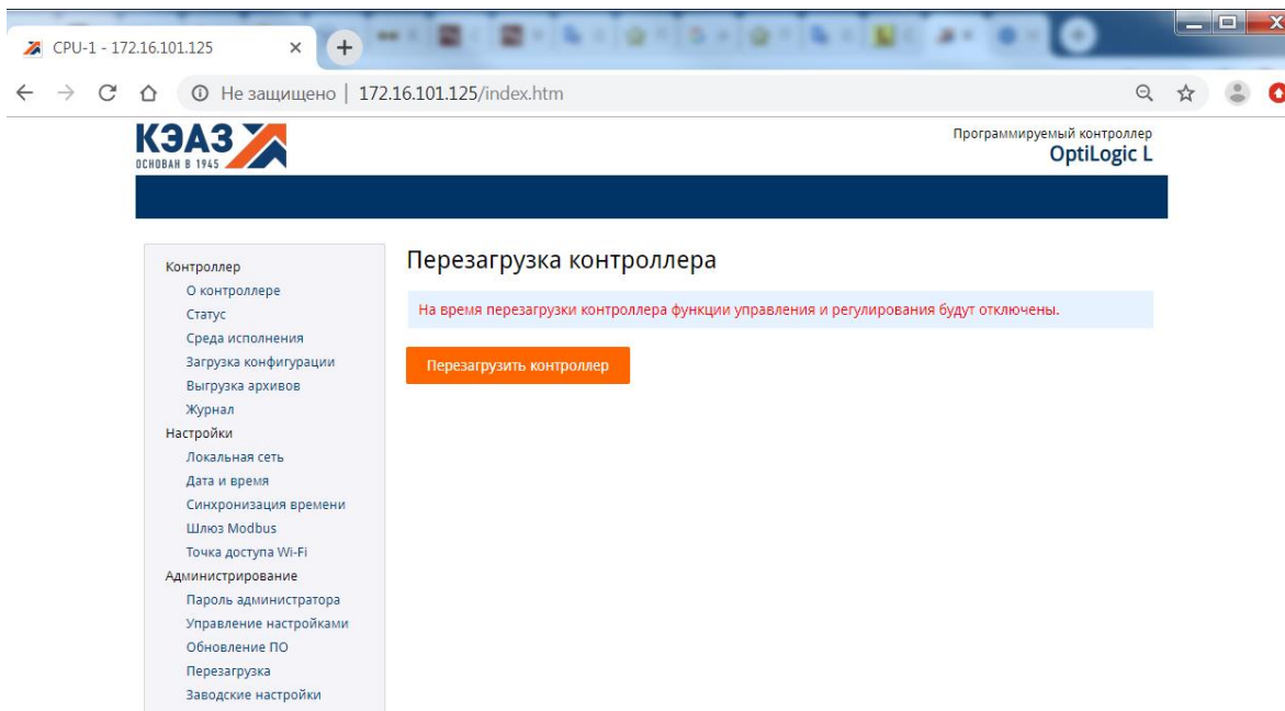
Рисунок 26 – Web-консоль, страница «Перезагрузка».
