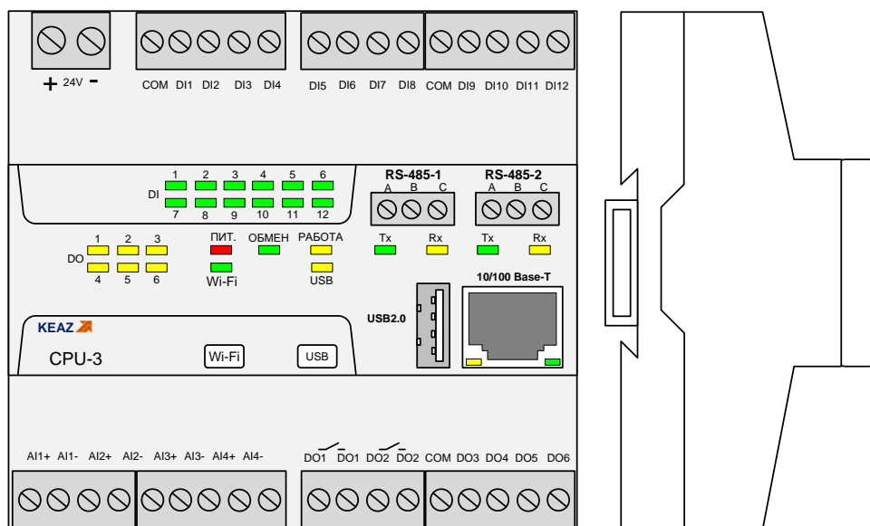
Рисунок 1 – Внешний вид и размеры модуля
