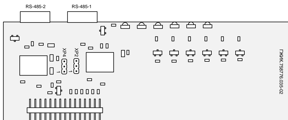
Рисунок 5 – Расположение перемычек XP2 и XP4
