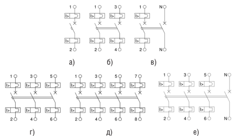
а) однополюсного; б) двухполюсного с двумя защищенными полюсами; в) двухполюсного с одним защищенным и нейтральным полюсами; г) трёхполюсного; д) четырёхполюсного с четырьмя защищенными полюсами; е) четырёхполюсного с тремя защищенными полюсами.
