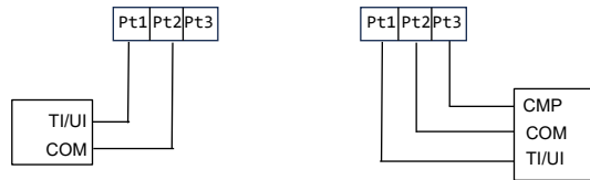
Выход NTC 10K 2-проводная схема
