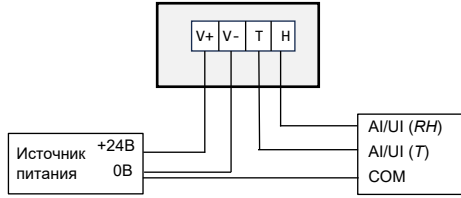
Схема подключения выходов влажности и температуры 0...10 В пост. тока
