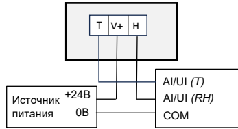
Схема подключения выходов влажности и температуры 4...20 мА
