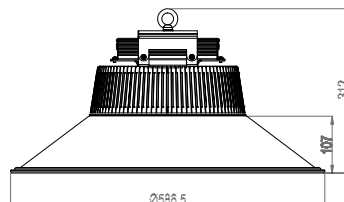
PHB SMD 200w 6500K + рефлектор 2855800 120° IP54
