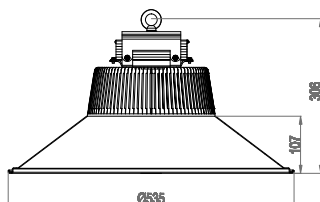
PHB SMD 100w 6500K + рефлектор 2850744 120° IP54 PHB SMD 150w 6500K + рефлектор 2850744 120° IP54
