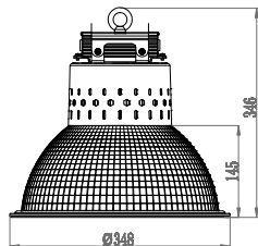
PHB SMD 50w 6500K + рефлектор 2850720 60° IP54 PHB SMD 70w 6500K + рефлектор 2850720 60° IP54
