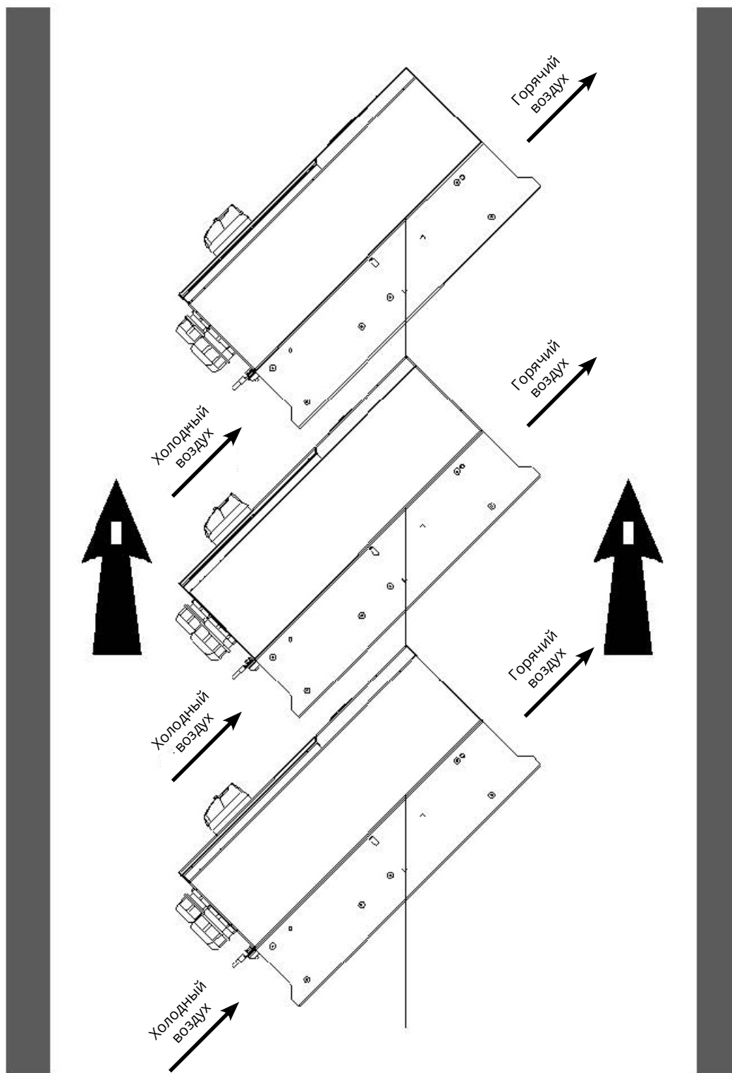
Рис 4.6 Наклонная установка
