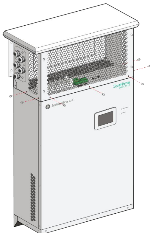
Рис. 5.5.3.1 Крепление влагозащитного комплекта IP31 к модулю АФГ
