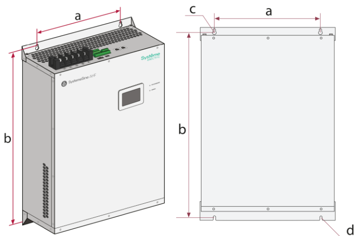
Рис. 5.5.2. Монтаж навесного модуля IP20
