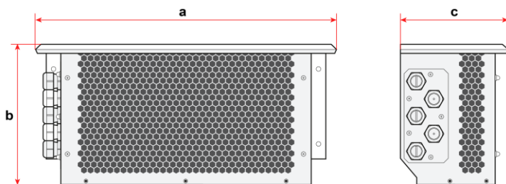
Рис. 3.6.3 Габаритные размеры влагозащитного комплекта IP31
