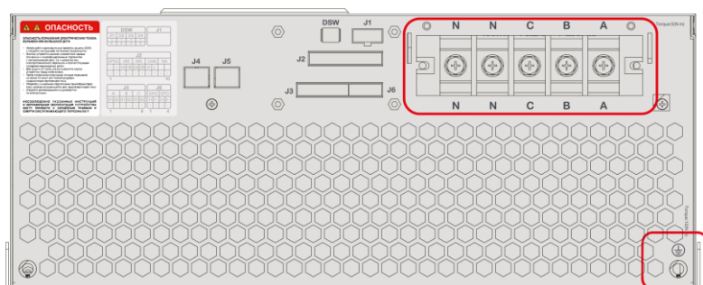
Рис. 6.2.2 Силовые клеммы питания стоечного модуля
