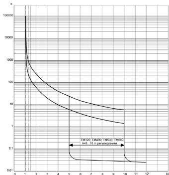
Рисунок 3 – Время-токовые характеристики выключателей OptiMat D630-ТМ320; OptiMat D630-ТМ400; OptiMat D630-ТМ500; OptiMat D630-ТМ630 с регулируемой уставкой срабатывания расцепителей короткого замыкания
