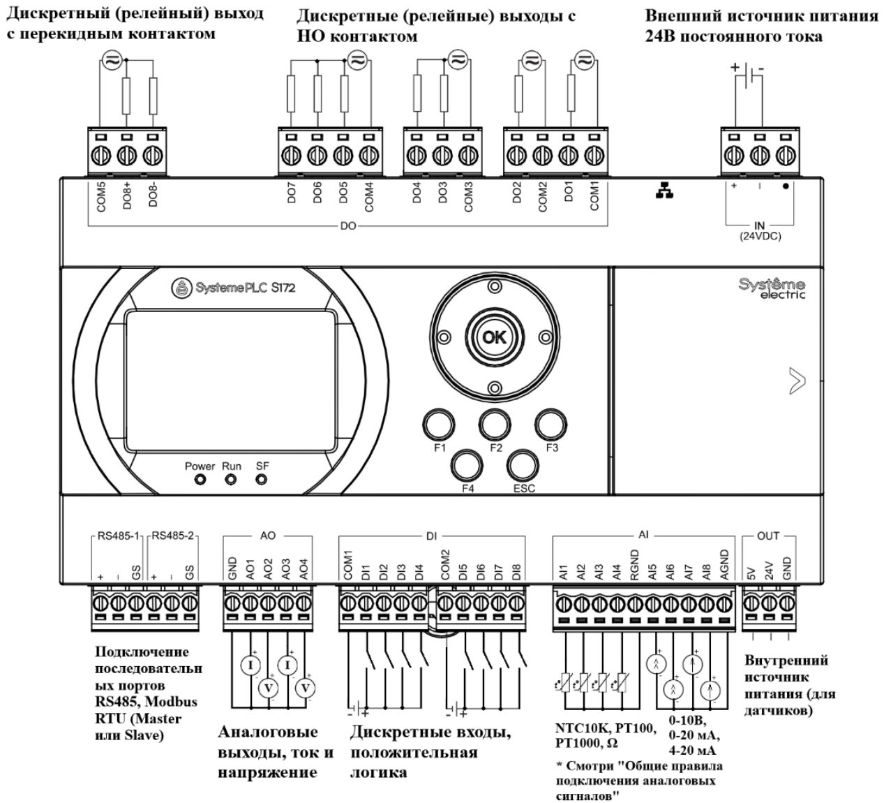
Рисунок 25 Схема подключений ПЛК SystemePLC S172 SM172PS11BDR
