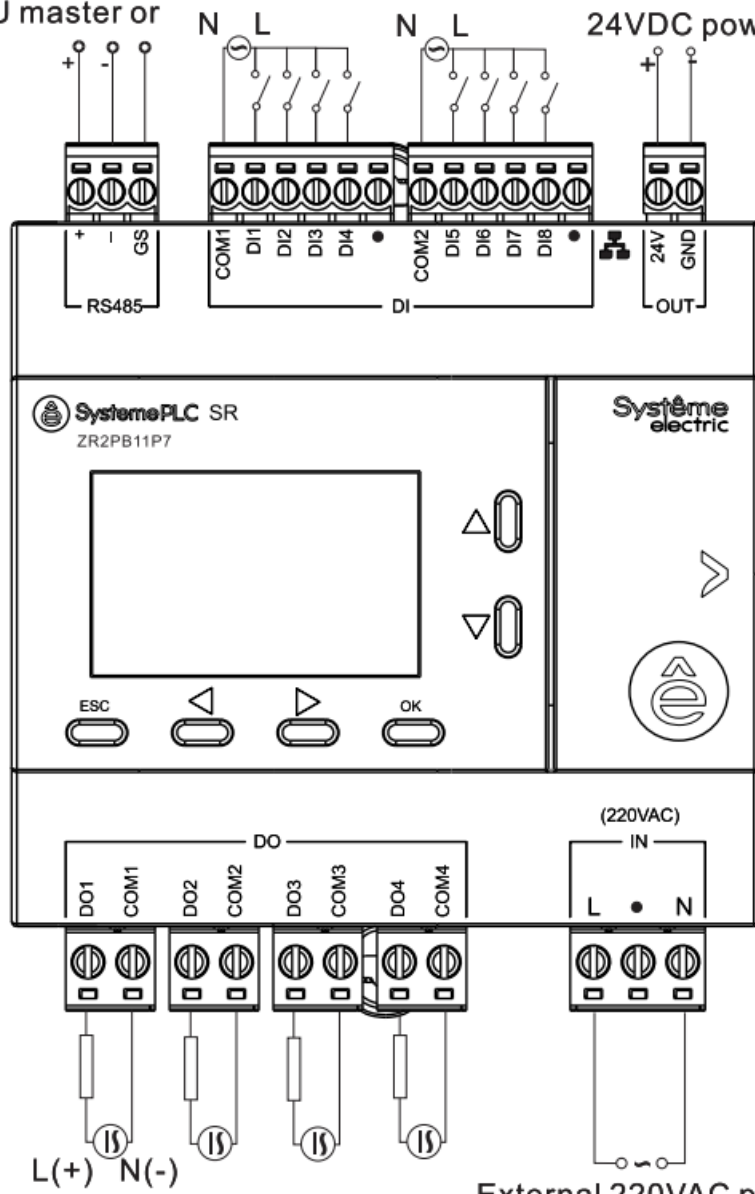
Рисунок 19 Схема подключений интеллектуального реле SystemePLC SR ZR2PB11P7
