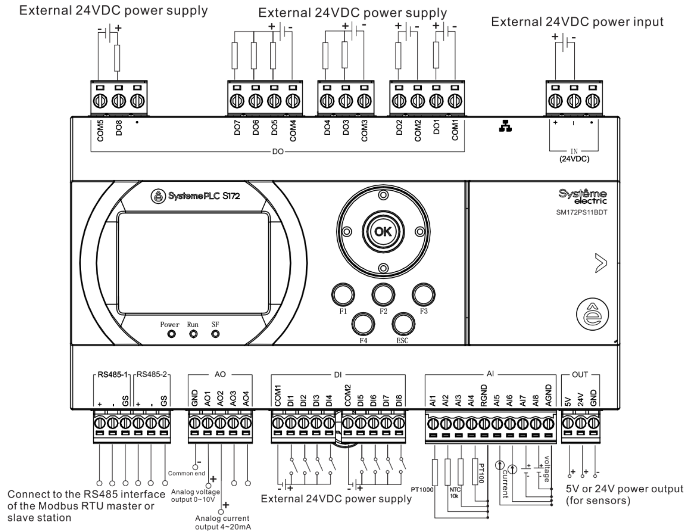
Рисунок 27 Схема подключений ПЛК SystemePLC S172 SM172PS11BDT
