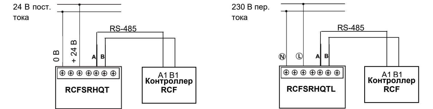
Схема подключения датчиков RCFSRHQT, RCFSRHQTL
