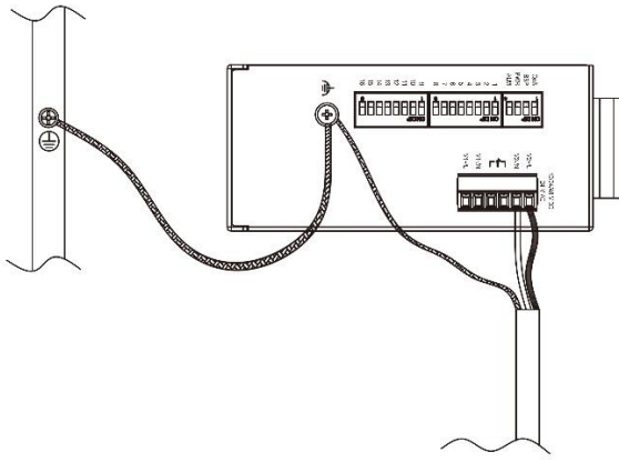
Рисунок 5 Примеры подключения питания коммутатора и концентратора
