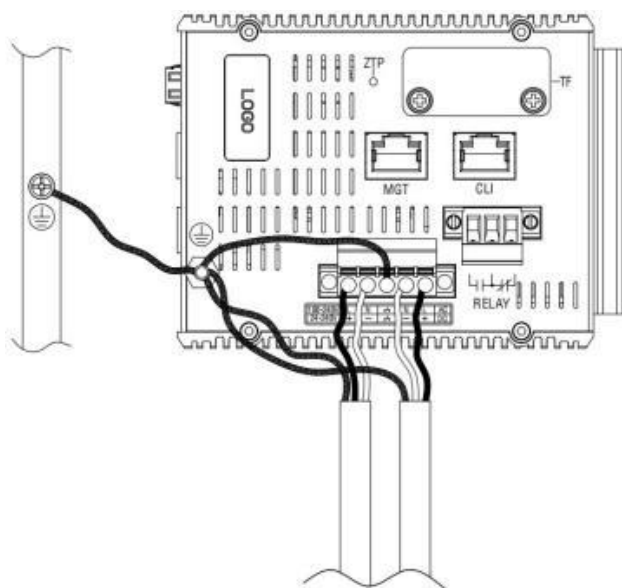
Рисунок 10 Заземление
