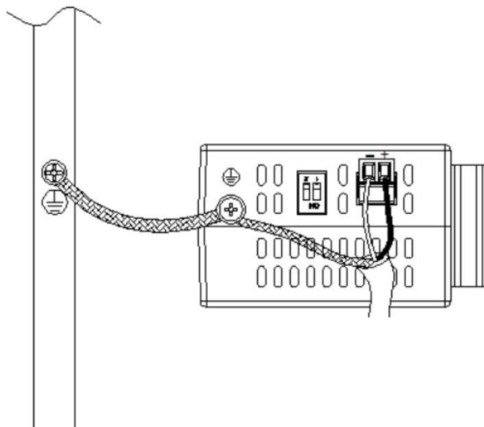
Рисунок 4 Схема подключения входного кабеля переменного/постоянного тока для модели с 8 портами
