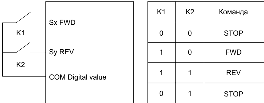
Рисунок 4-5 Двухпроводное управление тип 2
