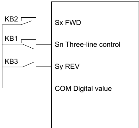
KB1: Кнопка «Стоп». KB2: Кнопка «Вперед». KB3: Кнопка «Назад».
