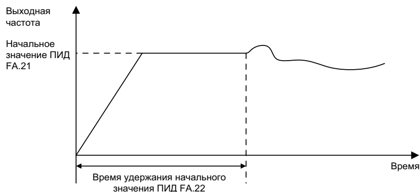
Рисунок 4-26 Алгоритм работы функции заполнения трубы
