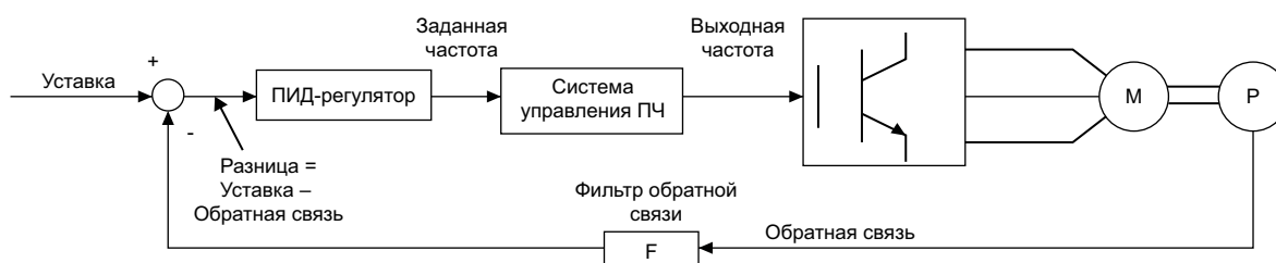
Рисунок 4-24 Блок-схема ПИД-регулирования
