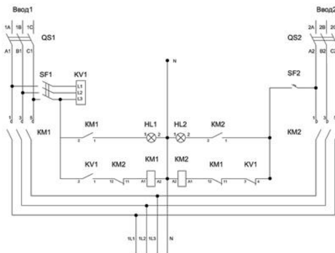
Рисунок 3. ЩАП-63, 73
