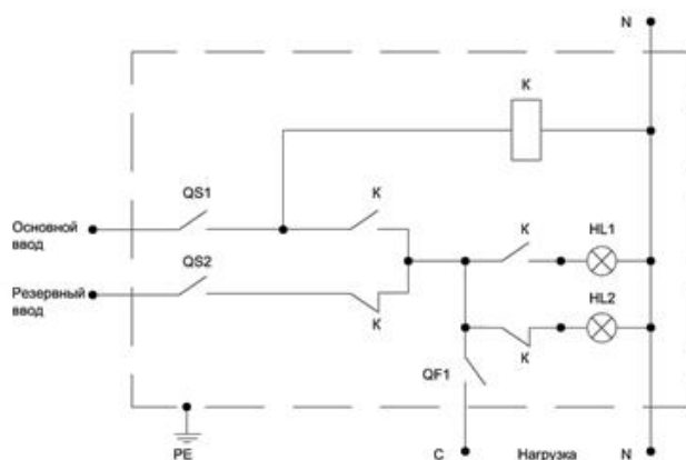
Рисунок 1. ЩАП-12
