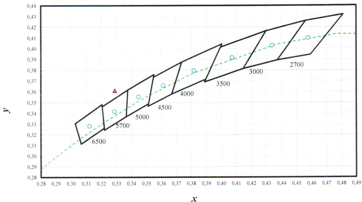
Диаграмма цветности x, y МКО-1931
