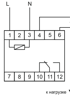
Рис. 2. Схема подключения.
