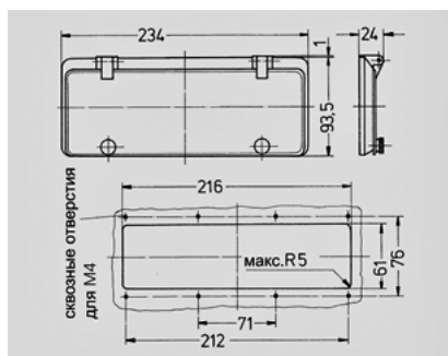
Чертеж 6 МВ 14 Размеры, мм.
