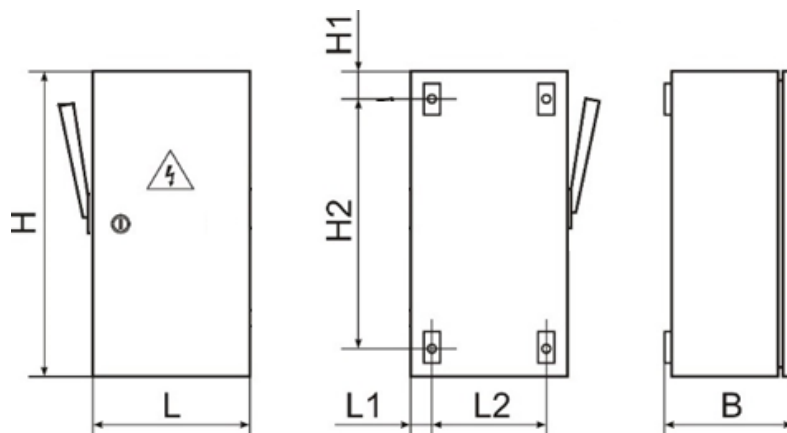
Общий вид и габаритные размеры ящиков силовых ЯРПП
