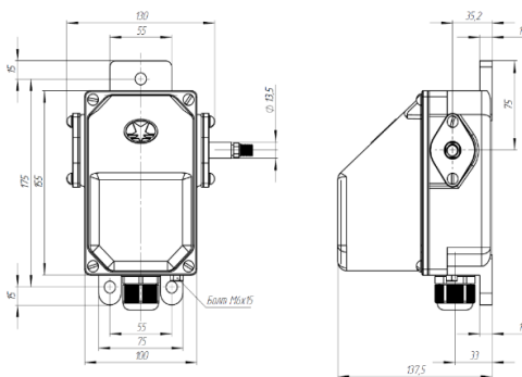
Рисунок 1. Общий вид, габаритные и установочные размеры путевых выключателей.
