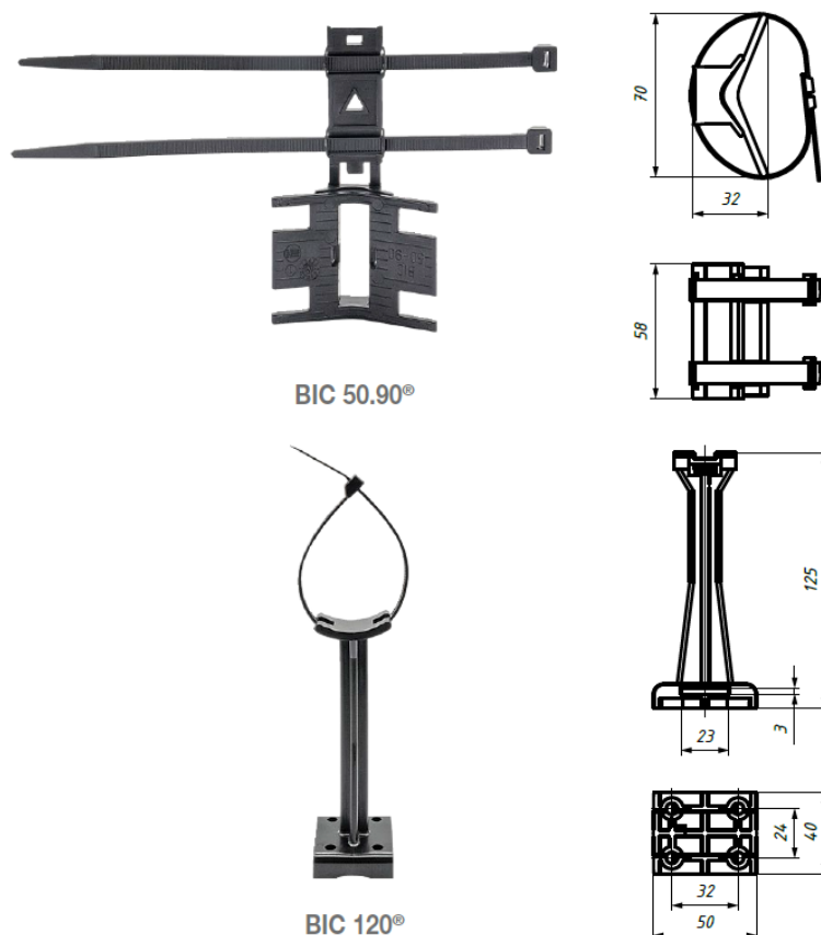
Рис. 1. Внешний вид дистанционных фиксаторов ВИС-15.50, ВИС-50.90, ВИС-120.
