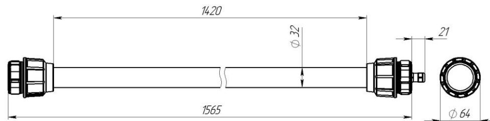
Рисунок 2 Светильник «L-line F».
