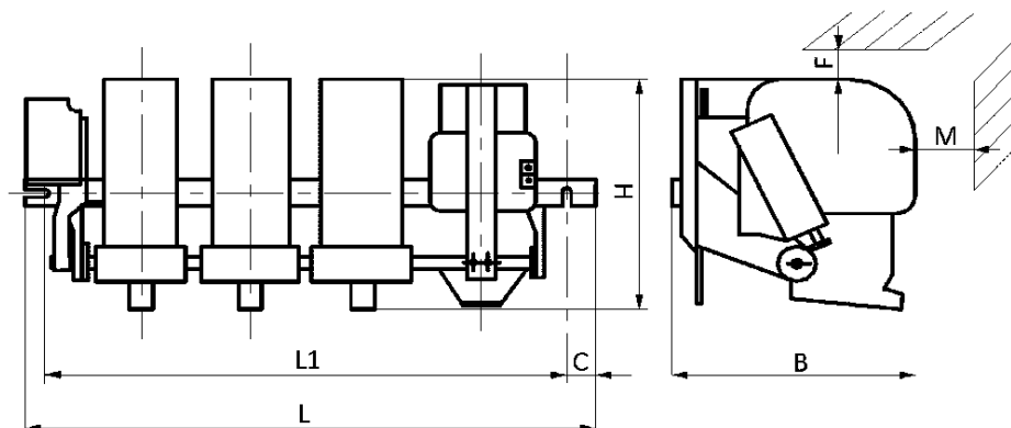
Рисунок 1. Габаритные и установочные размеры КТ-66х
