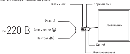
Рис.1. Схема подключения светильника к сети 220В.
