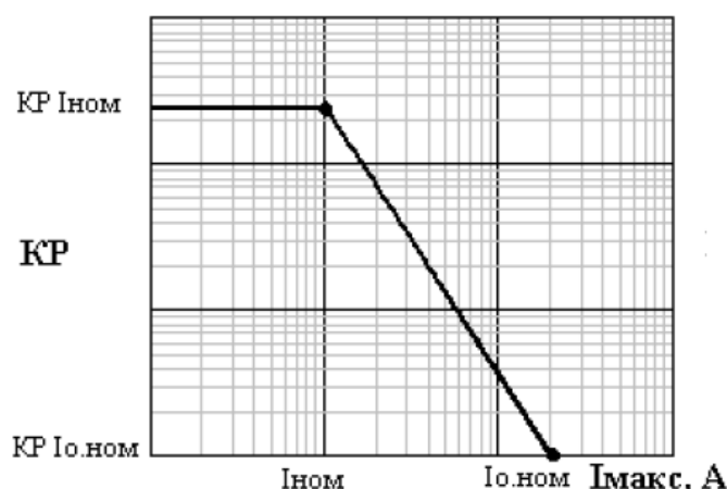
Рисунок 11 - Зависимость КР от максимального тока (в двойном логарифмическом масштабе)
