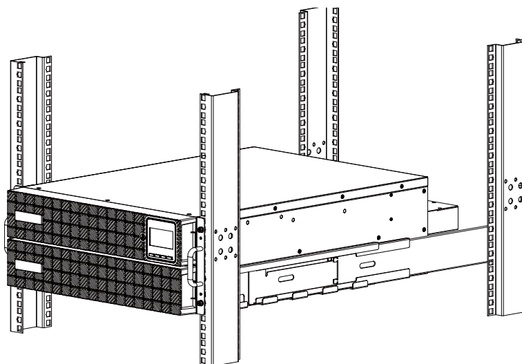
Рисунок 9-2. Установка ИБП
