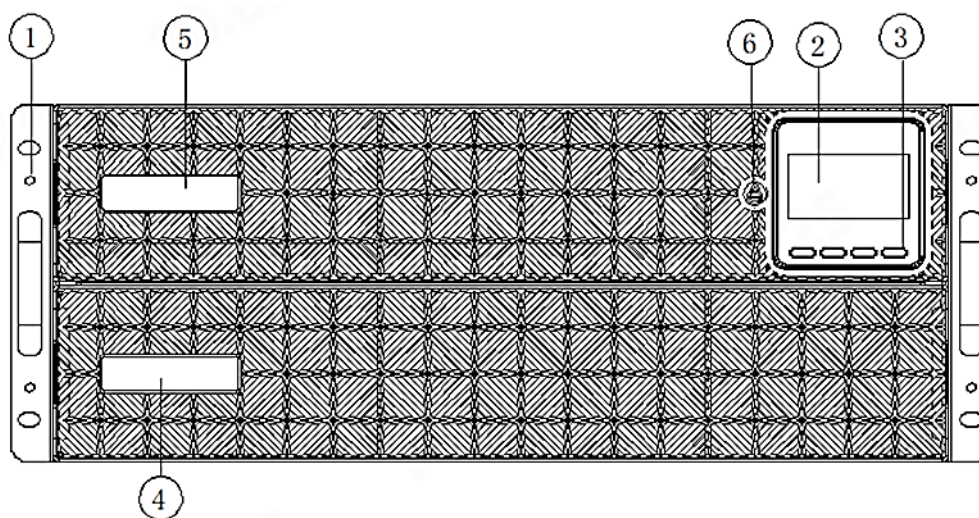
Рисунок 7-2. Вид спереди
