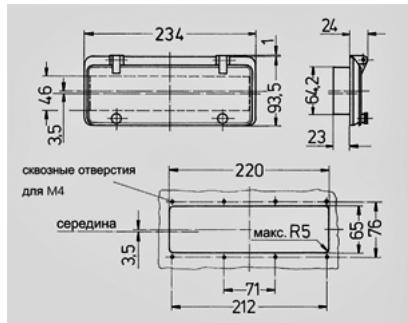
Чертеж 6 МВ 13 Размеры, мм.
